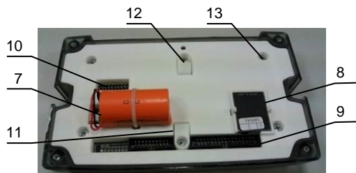
Рисунок 3.2 – Крышка
